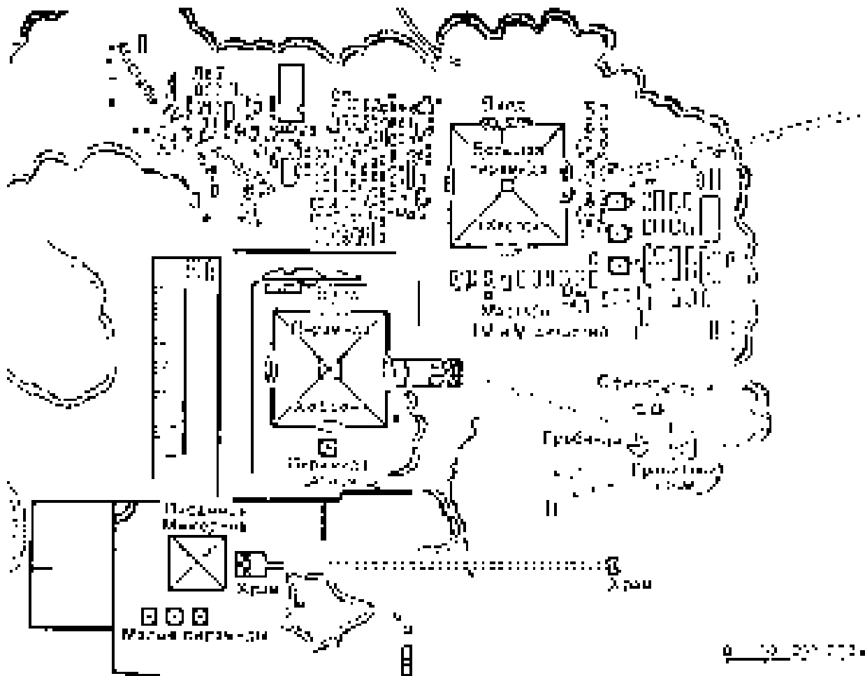
План части Гизэского некрополя.
